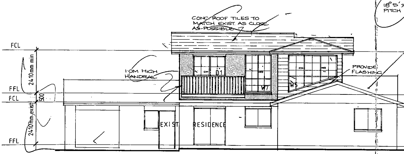
Elevation 3
